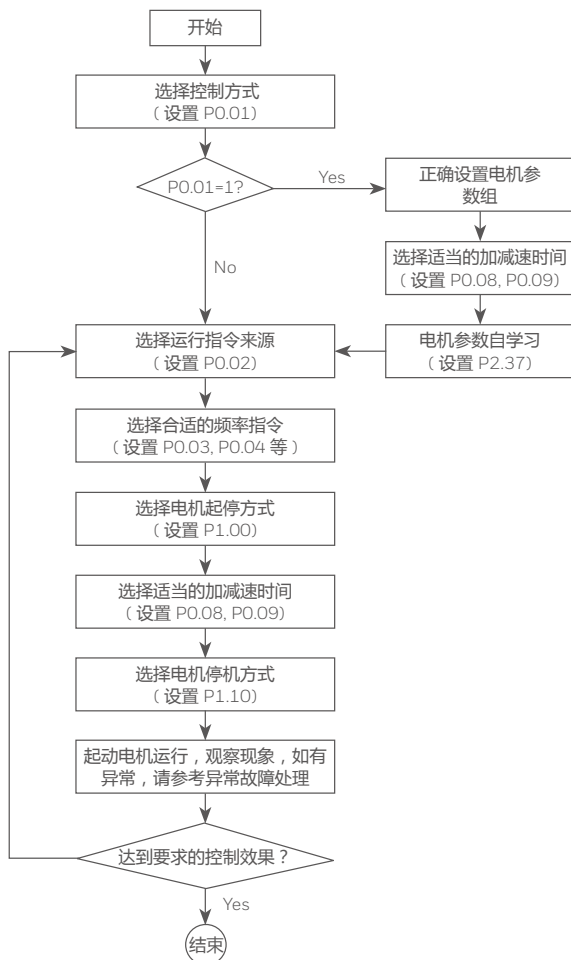
图 3-3 快速调试流程图
