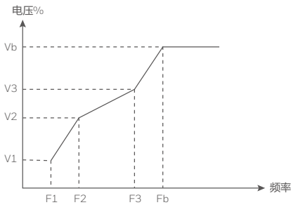
图 4-6 多点 V/F 曲线设定示意图
