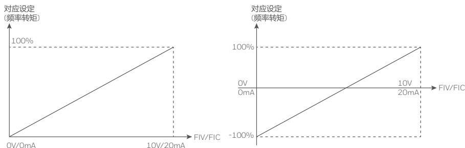
图 4-11 模拟给定与设定量的对应关系
