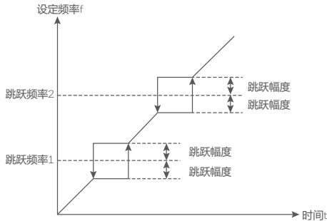
图 4-12 跳跃频率示意图
