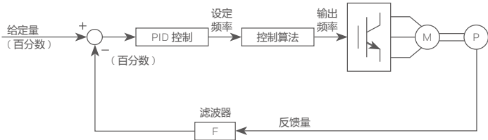
图 4-23 过程 PID 原理框图
