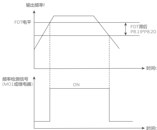
图 4-14 FDT 电平示意图
