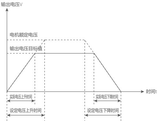
图 4-7 V/F 分离示意图
