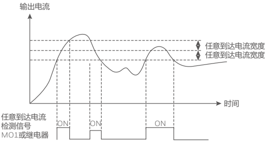
图 4-21 任意到达电流检测示意图
