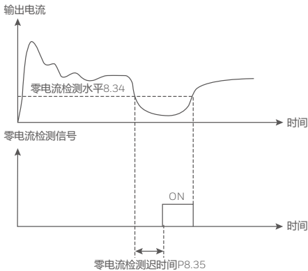
图 4-19 零电流检测示意图
