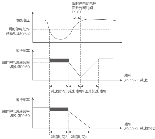
图 4-22 瞬时停电动作示意图
