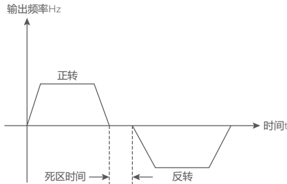
图 4-13 正反转死区时间示意图
