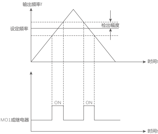
图 4-15 频率到达检出幅值示意图
