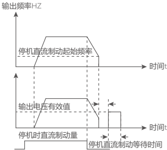
图 4-3 停机直流制动示意图
