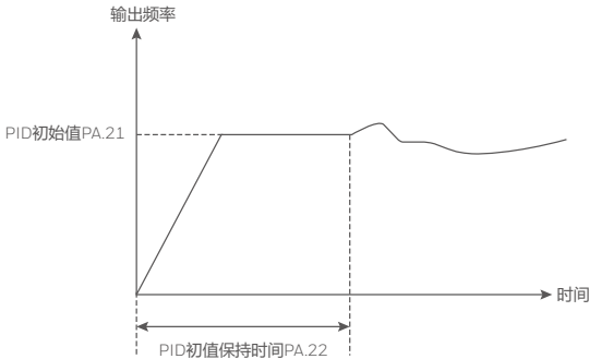
图 4-25 PID 初值功能示意图
