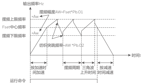
图 4-26 摆频工作示意图
