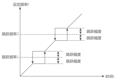
图 4-16 加减速过程中跳跃频率有效示意图
