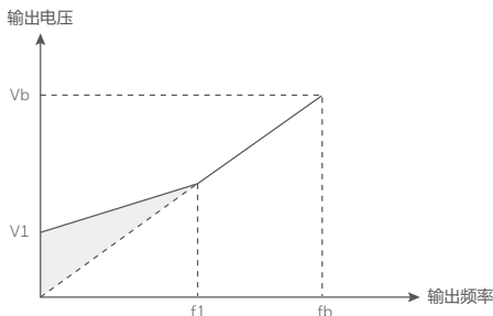
图 4-5 手动转矩提升示意图
