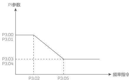
图 4-4 PI 参数示意图
