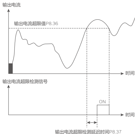
图 4-20 输出电流超限检测示意图
