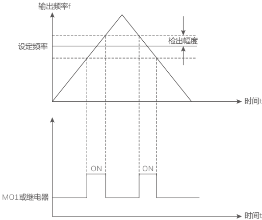
图 4-18 任意到达频率检测示意图
