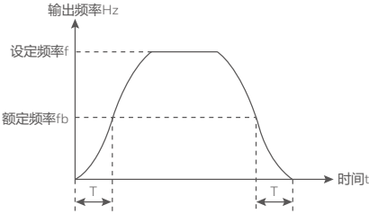
图 4-1 S 曲线加减速 B 示意图
