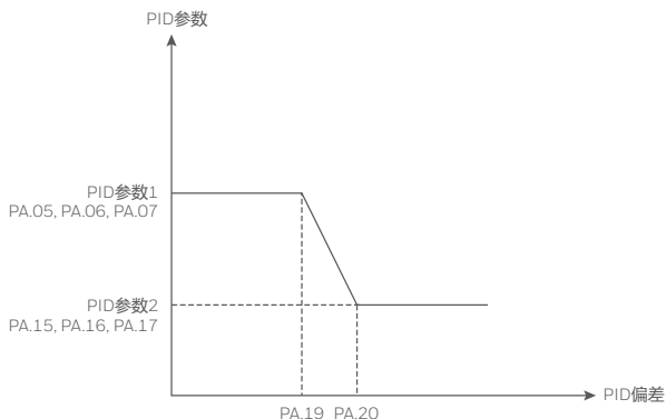
图 4-24 PID 参数切换
