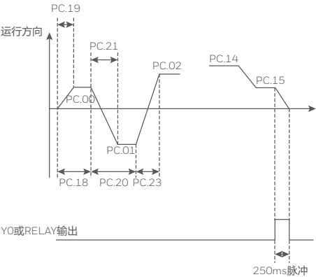
图 4-28 简易 PLC 示意图
