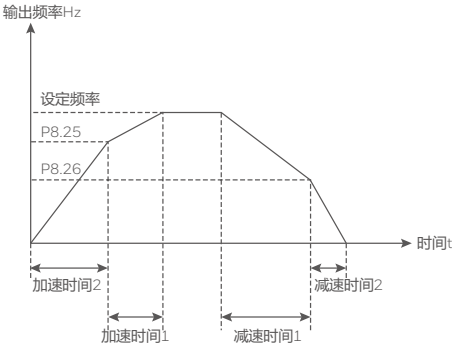
图 4-17 加减速时间切换示意图
