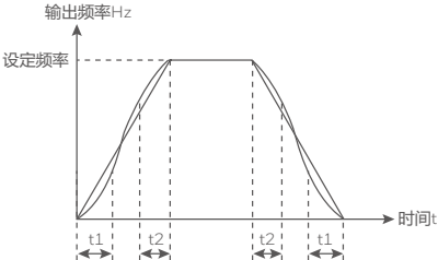
图 4-2 S 曲线加减速 A 示意图
