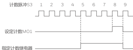
图 4-27 设定计数值给定和指定计数值给定示意图
