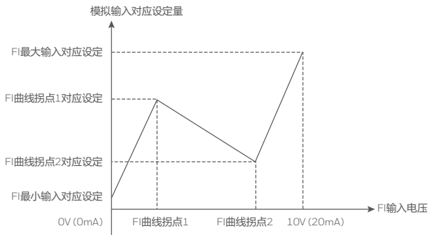
图 4-29 曲线 4 和曲线 5 示意图
